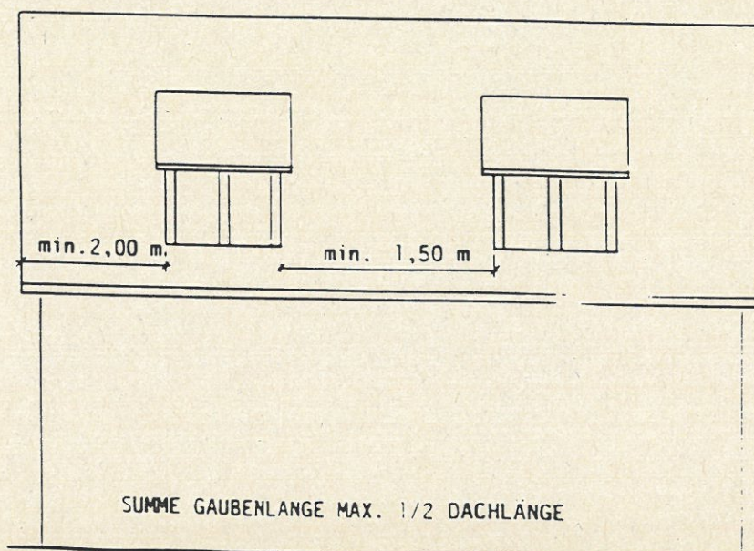
SCHLEPPGAUBEN
