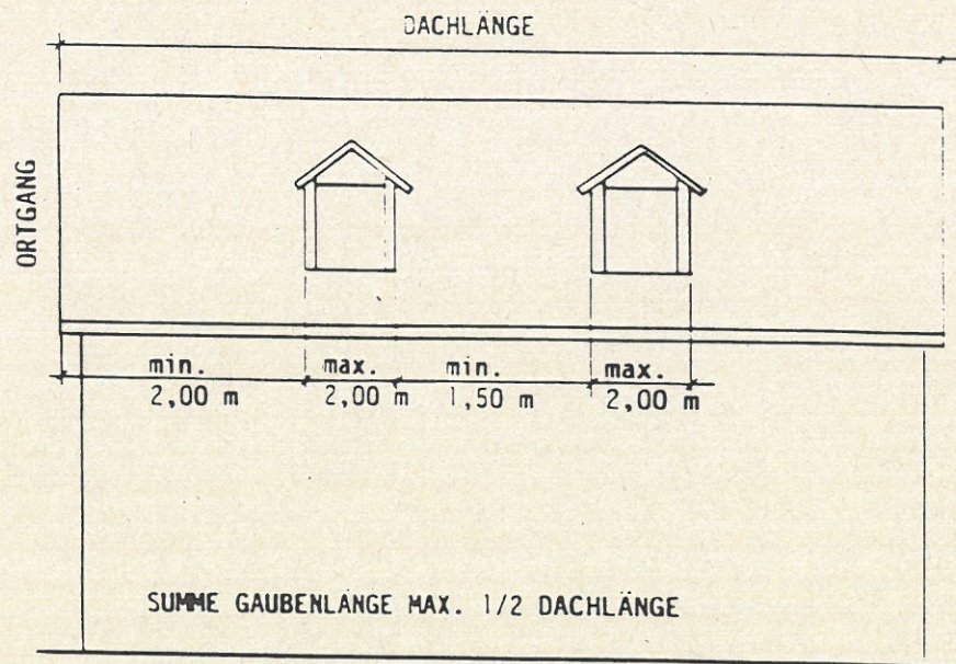
(giebelständige Gaube)
