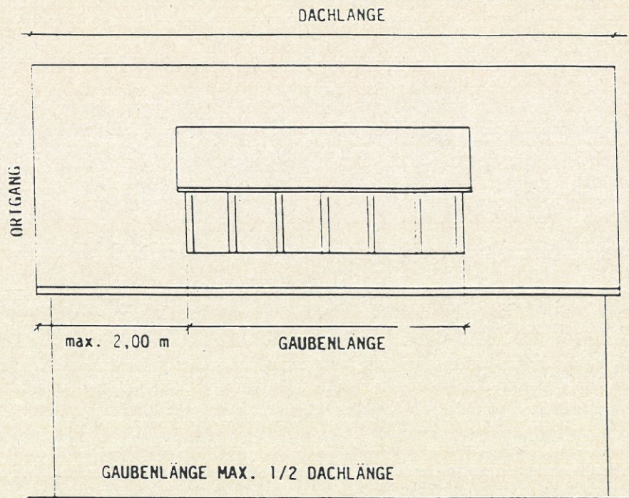
SATTELDACHGAUBE
