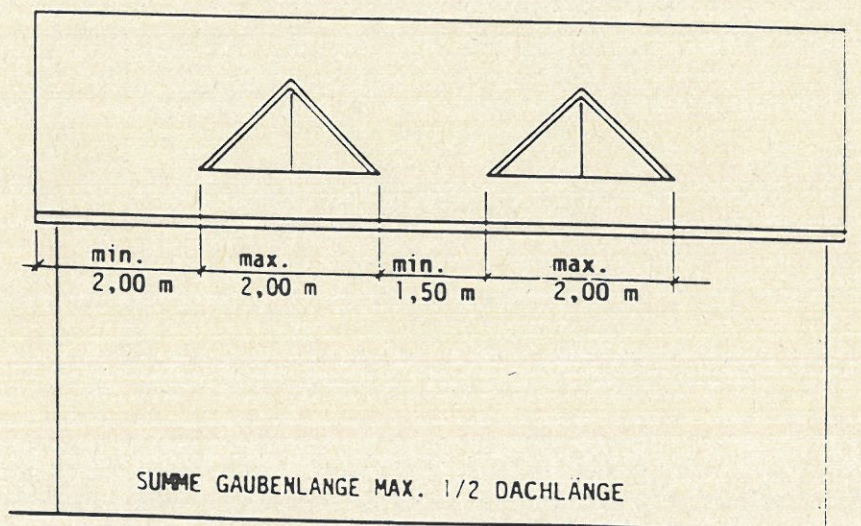
DREIECKSGAUBE
